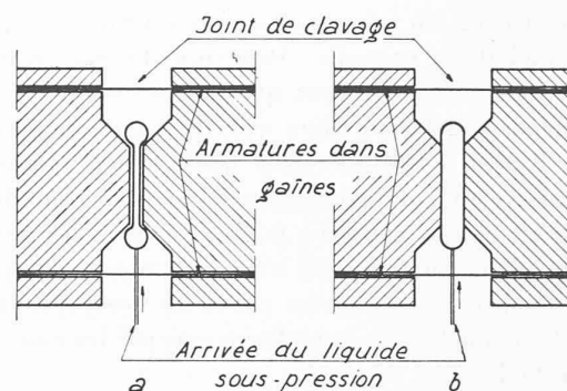
Fig. 4. — Vérin capsulaire : a) au repos ; b) en action.
