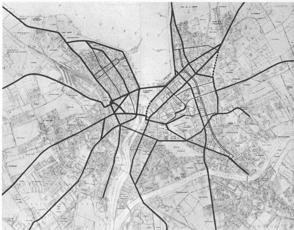
Fig. 8. — Réseau cohérent d'artères obtenu par les 4 transformations de quartiers proposées.
