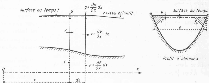
Fig. 5. — Petits mouvements non-permanents d'un liquide dans un canal découvert de profil variable.
