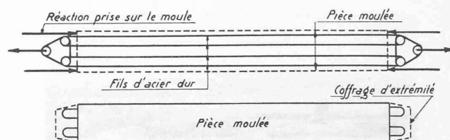
Fig. 8. — Précontrainte par moule individuel.
