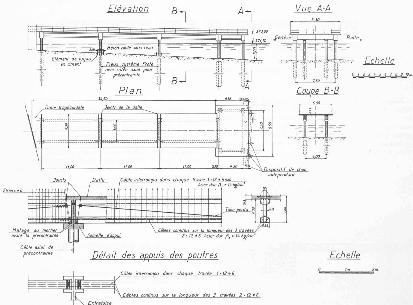
Fig. 3. — Plan, élévation et coupe du nouveau débarcadère. (Lire \beta_r < 14 \text{ t/cm}^2 ).
