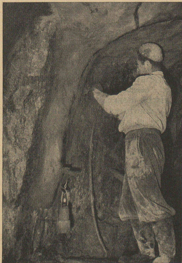
Forces motrices de l'Oberaar Etanchéité préalable de la galerie sous pression avec du BARRA Rapide U
