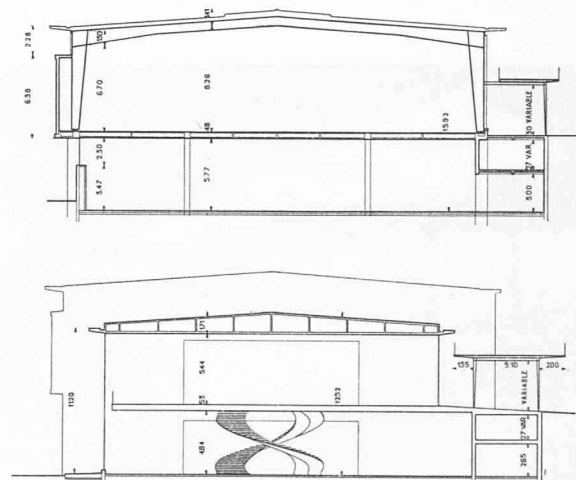
Fig. 5. — Coupes sur l'un des pavillons sud. Echelle 1 : 600.
