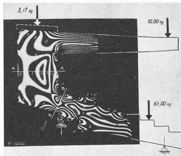
Fig. 14. — Modèle II : Lignes isochromes. ( \sigma_I - \sigma_{II} ) = const.
