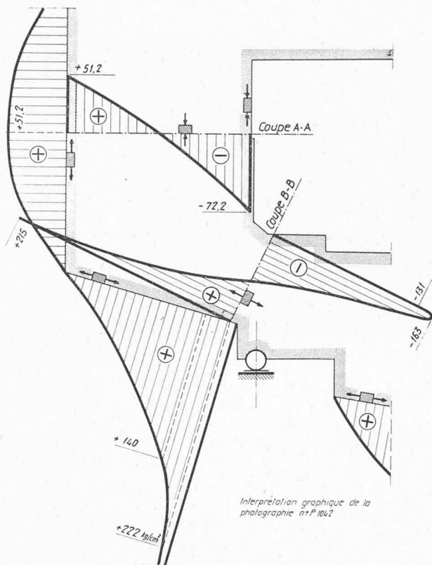
Fig. 8. — Modèle I: Contraintes en kg/cm² sur l'ouvrage. a) Contraintes parallèles aux bords (contraintes principales). b) Contraintes normales dans les sections A-A et B-B.
