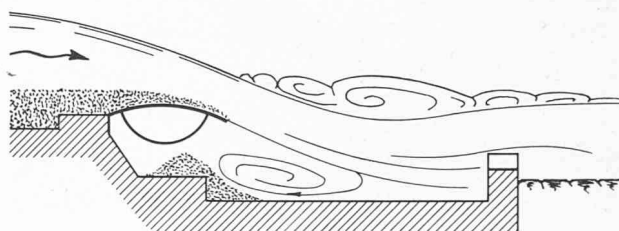
Fig. 8. — Engrèvement du radier, d'après M. Fischer [2].
