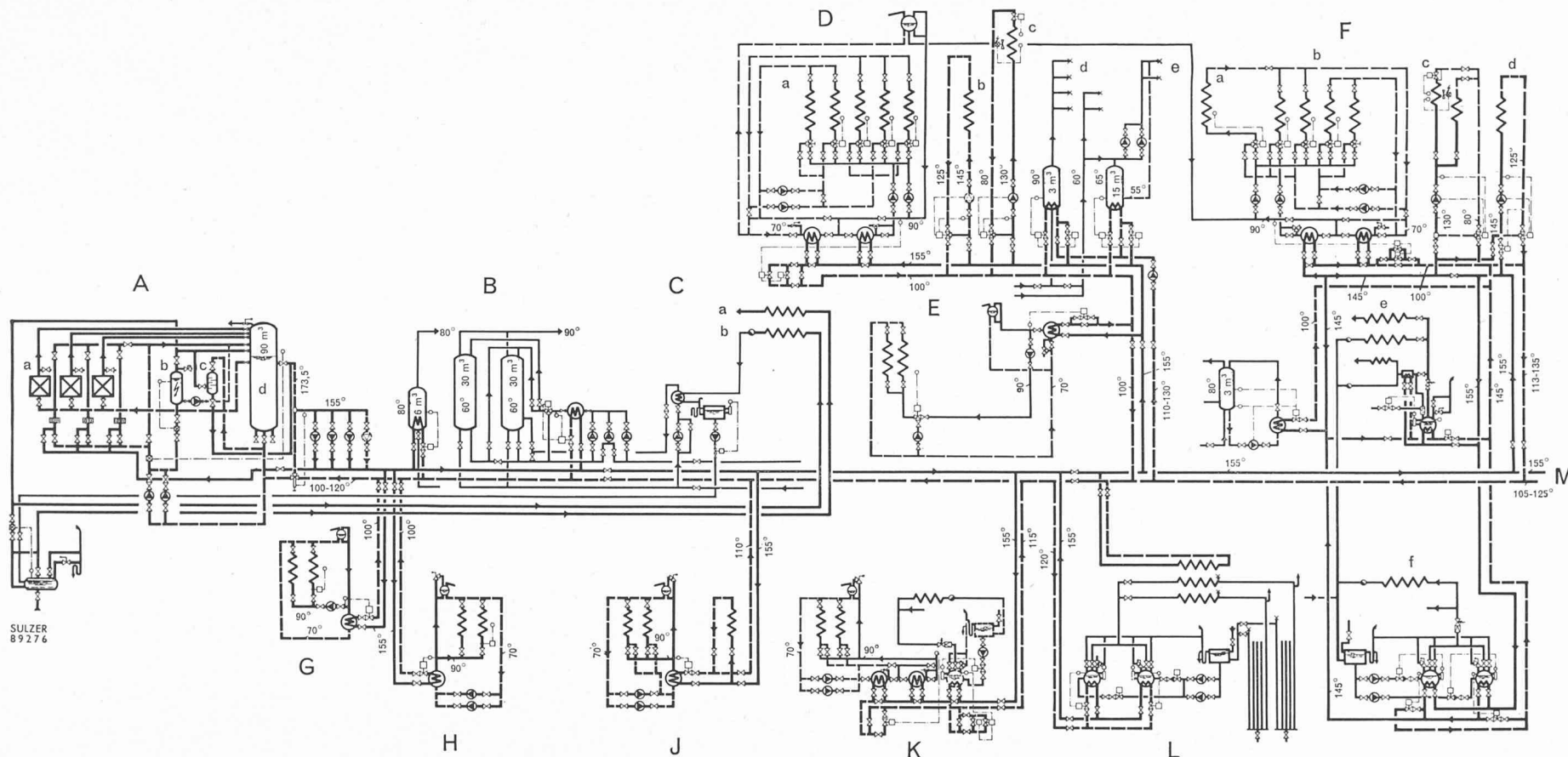
Fig. 5. — Schéma thermique.
