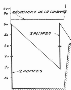
Fig. 11. — Ligne piézométrique, quatre pompes, fuel B, après un arrêt de quinze heures, débit environ 20 m³/h.
