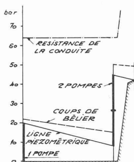
Fig. 9. — Ligne piézométrique et coups de bélier, trois pompes avec fuel B, débit 82 m³/h.
