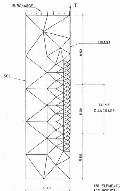
Fig. 9. — Réseau des éléments finis.
