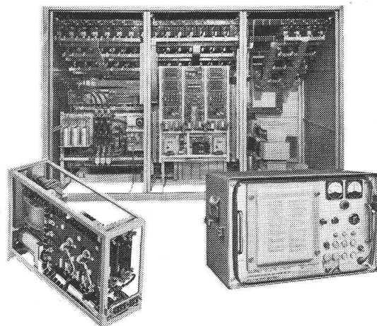
Onduleur dans tiroir 19".
