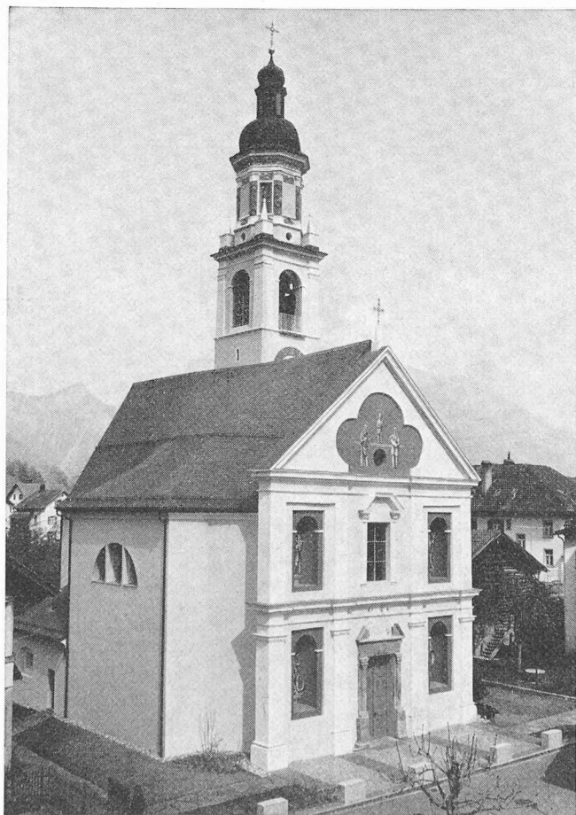
Fig. 9. — Eglise de Rhäzuns. Assèchement électro-osmotique des murs exécuté en 1968. (Photo C. Guler, Thusis.)
