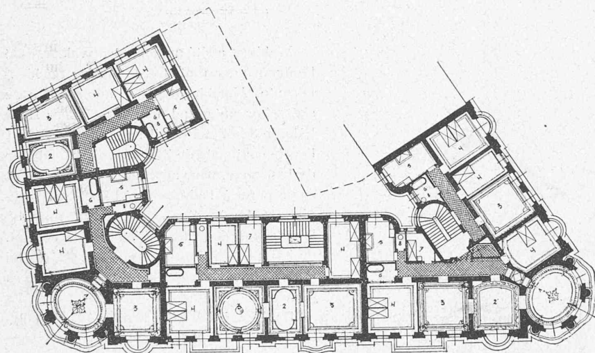
Plan des I er , II me et III me étages.
