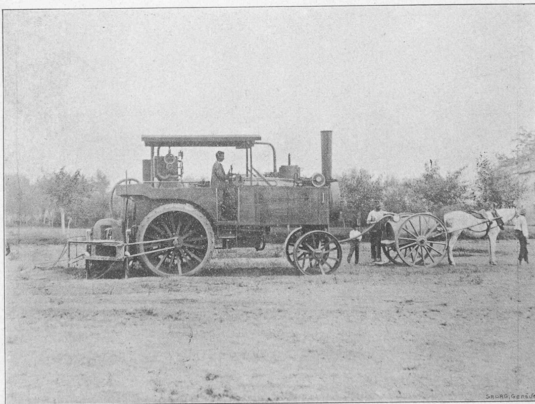
Fig. 4. — Laboureuse à vapeur s'approvisionnant d'eau en service.
