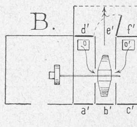
Fig. 17. — Refoulement de l'air dans le tunnel à pression double.
