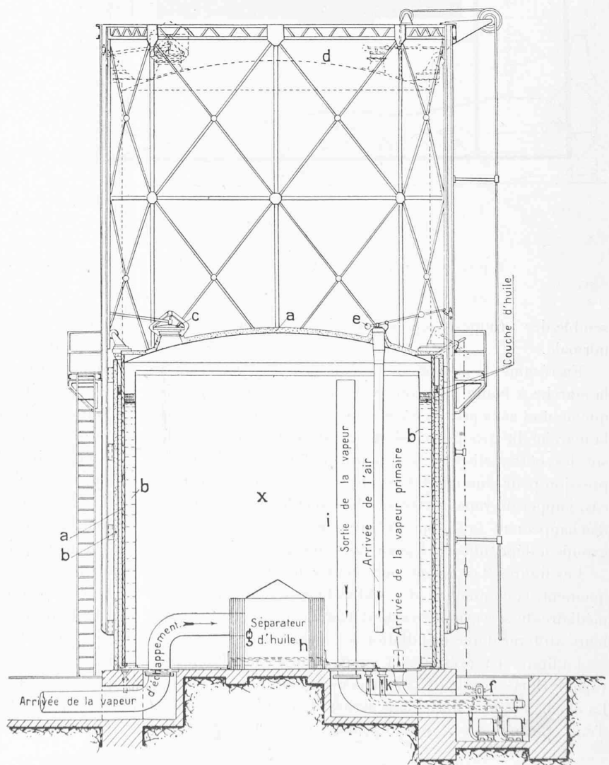
Fig. 4. — Accumulateur Harlé-Balcke.
