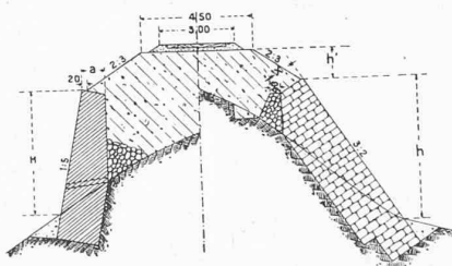
Type d'assise avec enrochement. a = 0,6 + 0,06 H. Mur à mortier avec avant-perré. x = 0,4 + 0,1 h + 0,5 h' \geq 0,7. Murs sous remblai. — 4 : 300.
