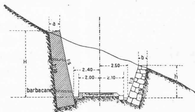
En maçonnerie à mortier. a = 0,60 + 0,06 H. En maçonnerie sèche. b = 0,60 + 0,05 h. Murs de revêtement. — 1 : 300.
