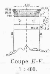
Fig. 6. — Pont sur la Drance.
