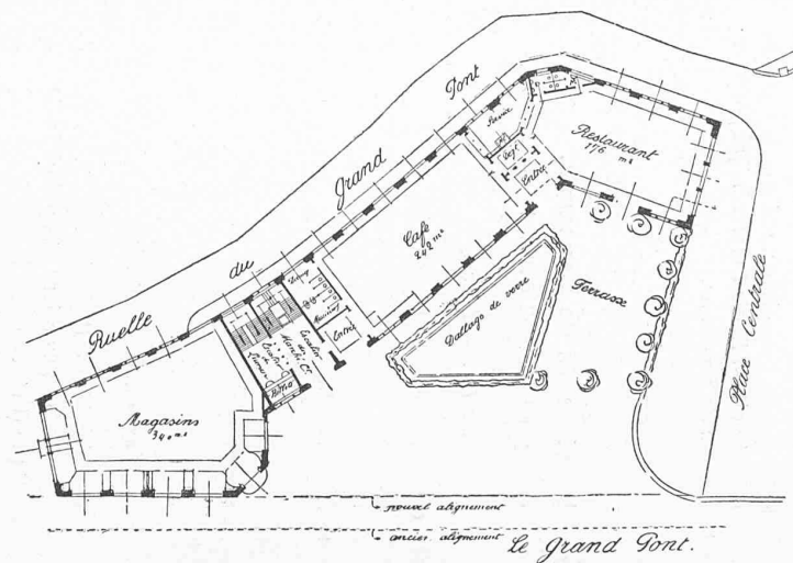
Plan au niveau du Grand-Pont — 1 : 800.
