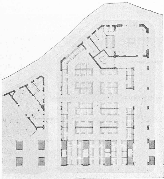
Plan de l'entresol — 1 : 800.
