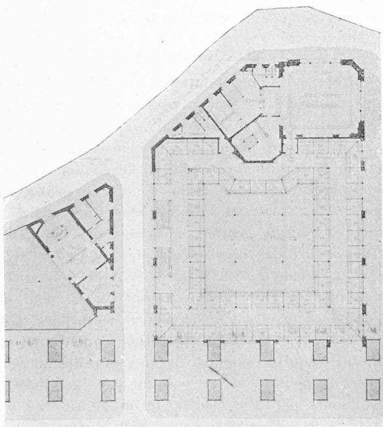
Plan du rez-de-chaussée inférieur — 1 : 800.
