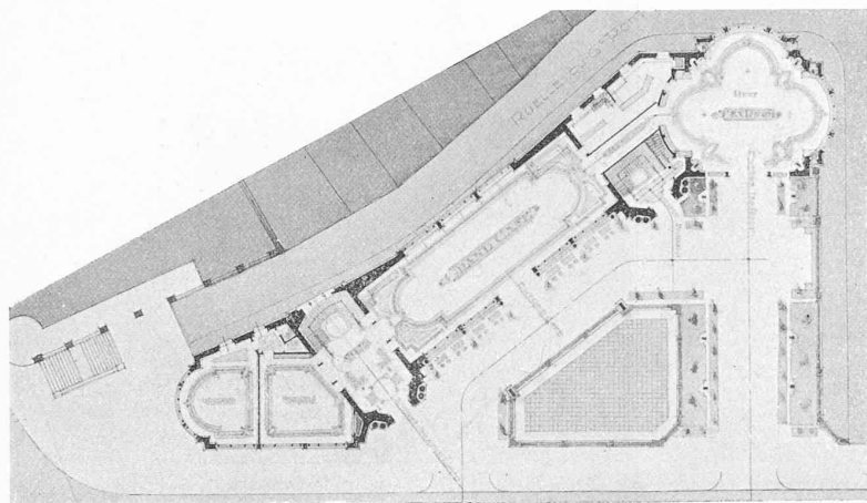
Plan au niveau du Grand-Pont — 1 : 800.
