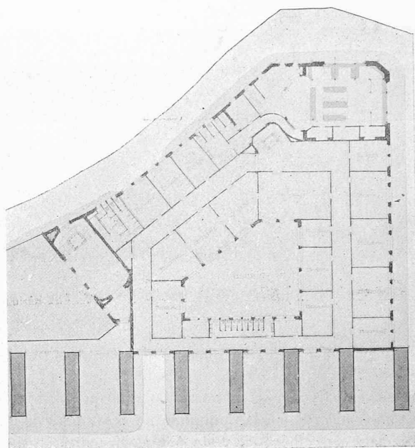
Plan de l'étage — 1 : 800.
