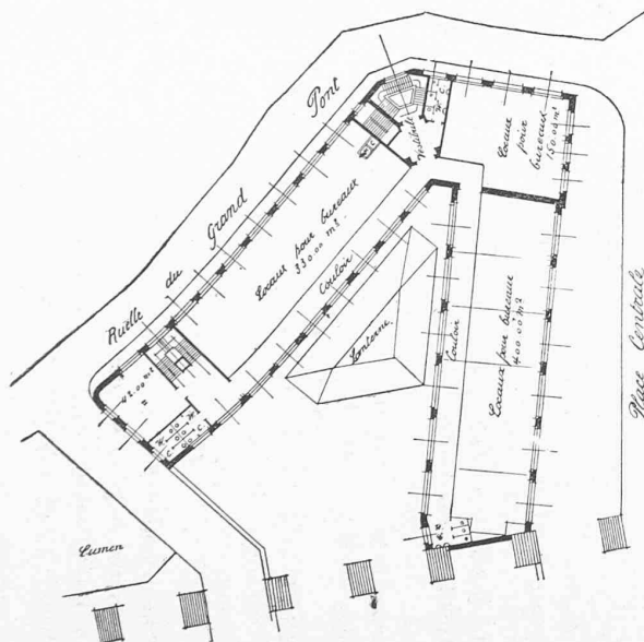
Plan du 1 er étage. — 1 : 800.
