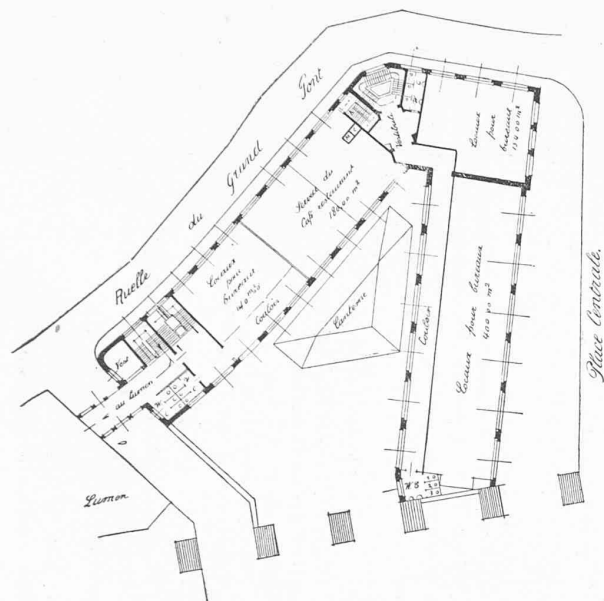
Plan du 11 me étage — 1 : 800.
