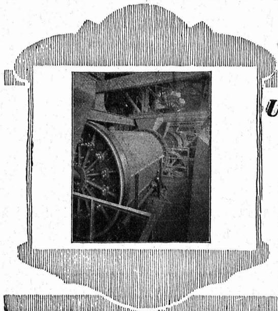
Concasseur automobile
