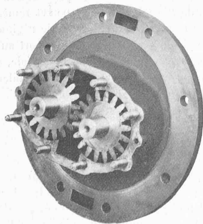
Fig. 11. — Pompe à engrenages destinée aux petits régulateurs.
