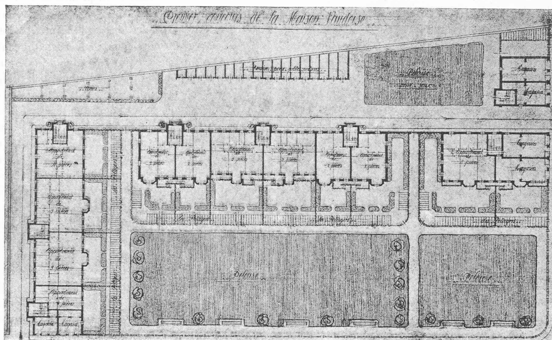
Plan général. — 1 : 800.
