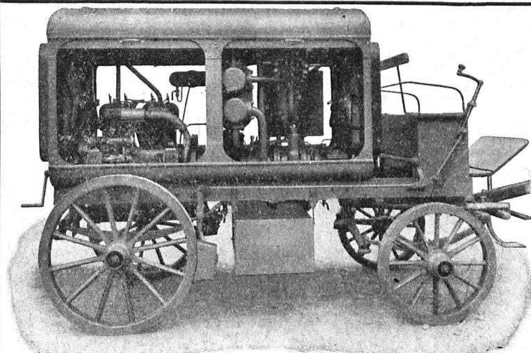
Moto-Compressur sur char.
