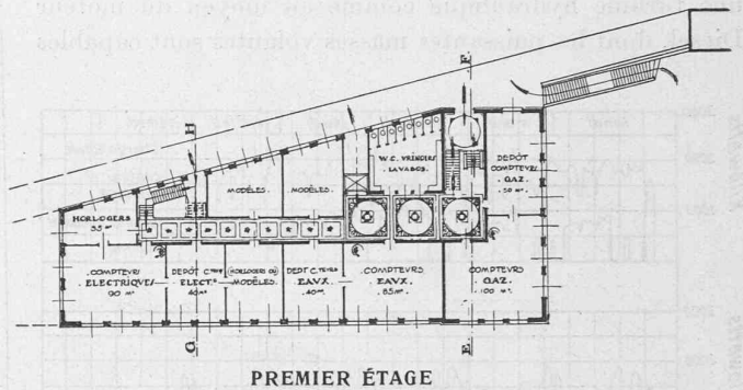
PREMIER ÉTAGE
