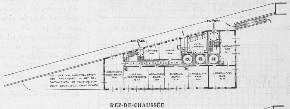
REZ-DE-CHAUSSÉE
