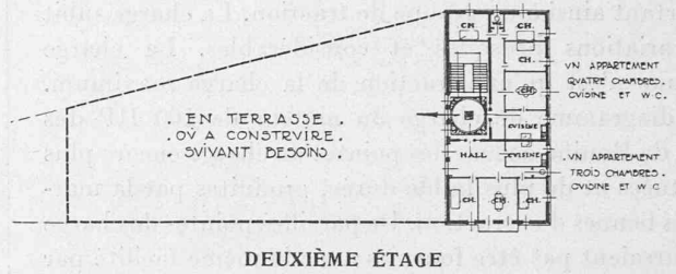
DEUXIÈME ÉTAGE
