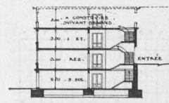
COUPE G-H
