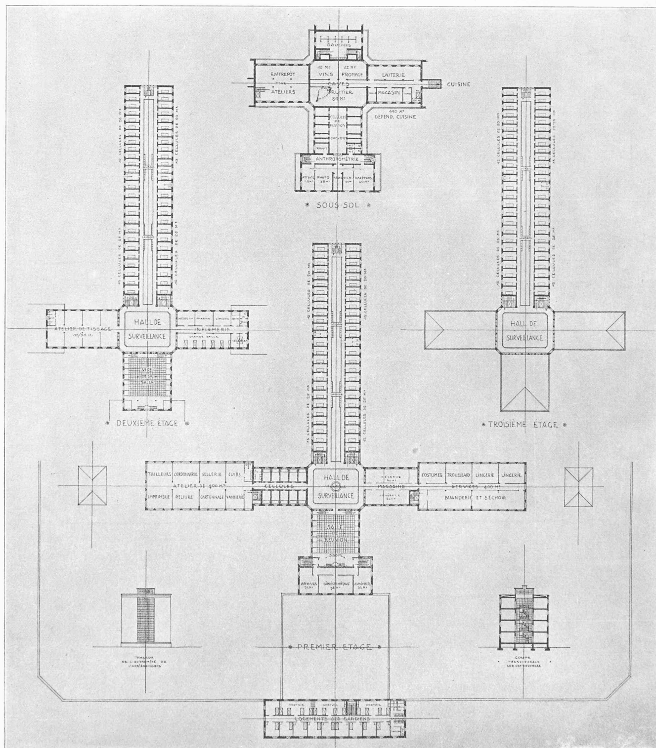
Plan du sous-sol, du 1 er , du II me et du III me étage. — 1 : 1000.
