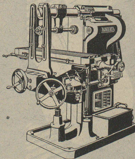
FRAISEUSE - WANDERER
