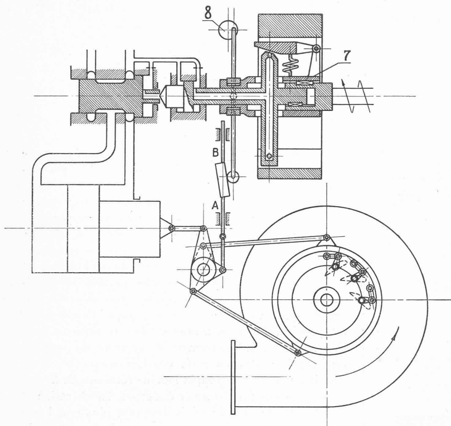
Fig. 10. — Ensemble schématique du régulateur.
