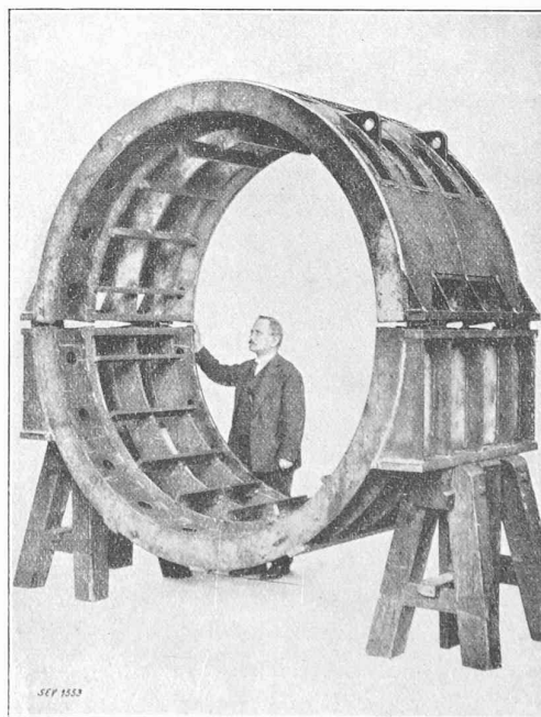
Fig. 17. — Carcasse d'un alternateur de 3800 kVA, Ateliers de Sécheron.
