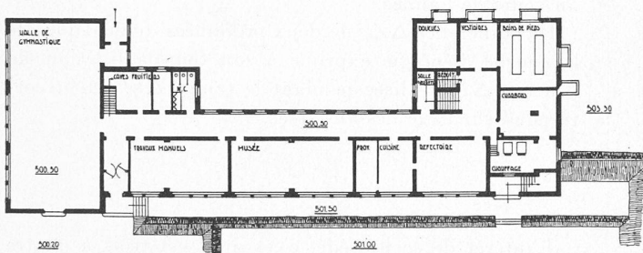
Plan du sous-sol. — 1 : 800.
