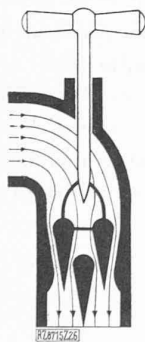
Fig. 2. — Robinet « insonorisé ».
