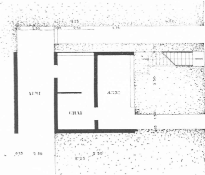
Rez-de-chaussée
