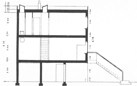
Coupe
