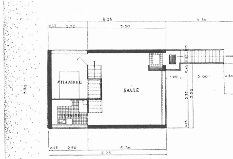
1er étage
