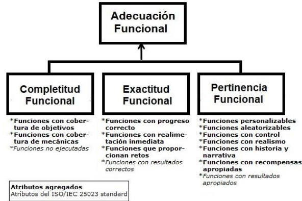
Fig. 2. Característica Adecuación Funcional: sub-características y atributos
