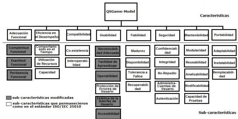
Fig. 1. QSGame-Model
